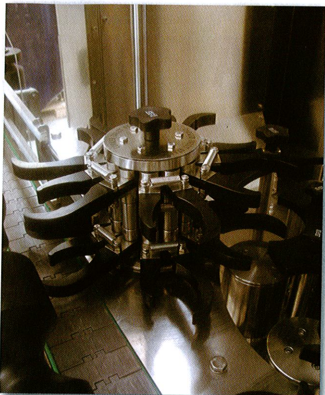
Gai France, médaille d'argent, vis et étoiles universelles automatiques pour l'embouteillage. L'étoile permet de traiter des bouteilles de diamètres de 60 à 115 mm, par un jeu de deux pinces sur le corps et sans modification de l'outillage. Stand 1 B 33
